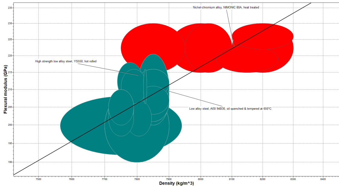
Figura 5: Diagrama de CES Edupack Para acero elegido para los cinces.
